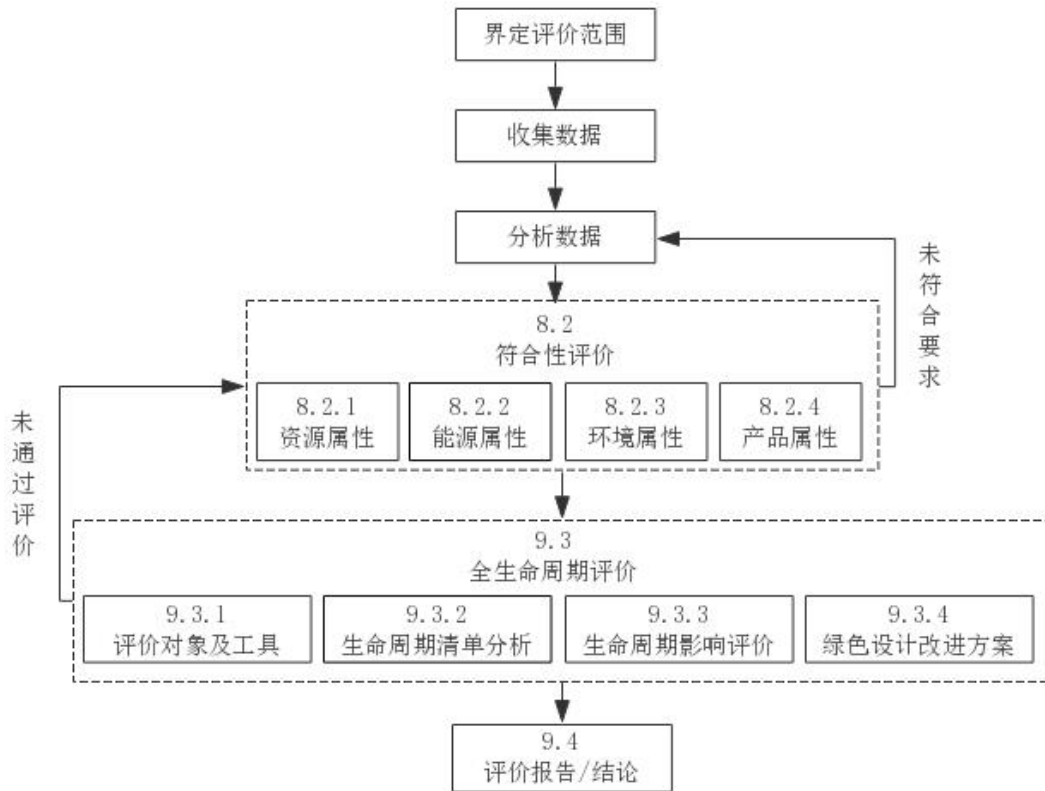
图1 一体机绿色设计评价流程
